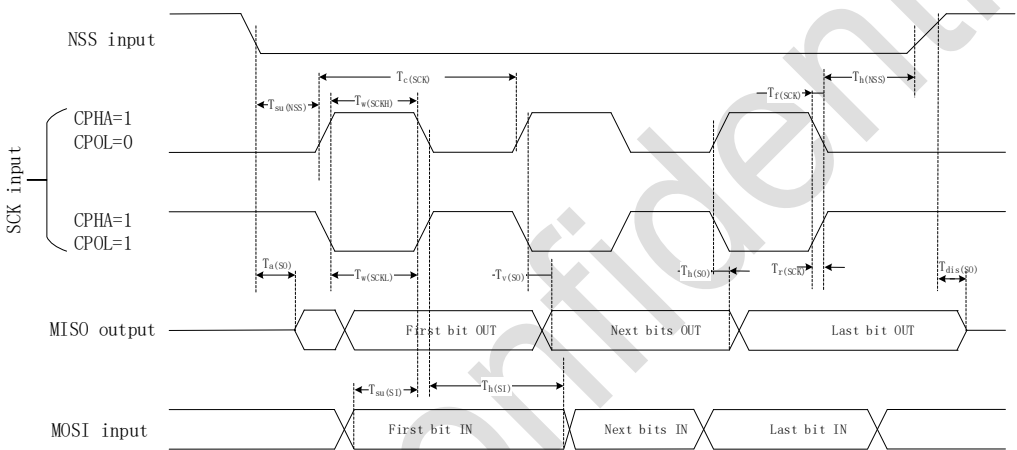
图 5-5 SPI 时序图 – 从机模式，CPHA = 1
